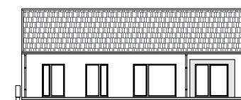
ELEWACJA OGRODOWA
